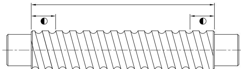
Fig 1.10.5 Harden Area
